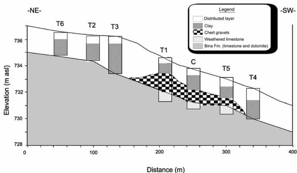
6 חתך סכמתי של הגיאומורפולוגיה בשטח C, מבט לדרום
