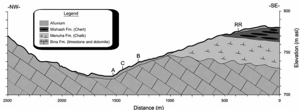
4 חתך סכמתי של הגיאולוגיה הכללית באזור עמק רפאים, מבט לצפון
